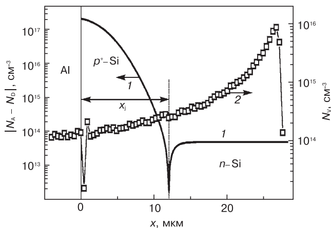
Рис. 1. Рассчитанные профили: распределения модуля разности концентраций акцепторов и доноров |N_A - N_D| в исходном диоде (1) и распределения первичных вакансий, образованных при облучении диодов ионами криптона с энергией 250 МэВ (2). Флюенс облучения \Phi = 10^8 \text{ см}^{-2}
