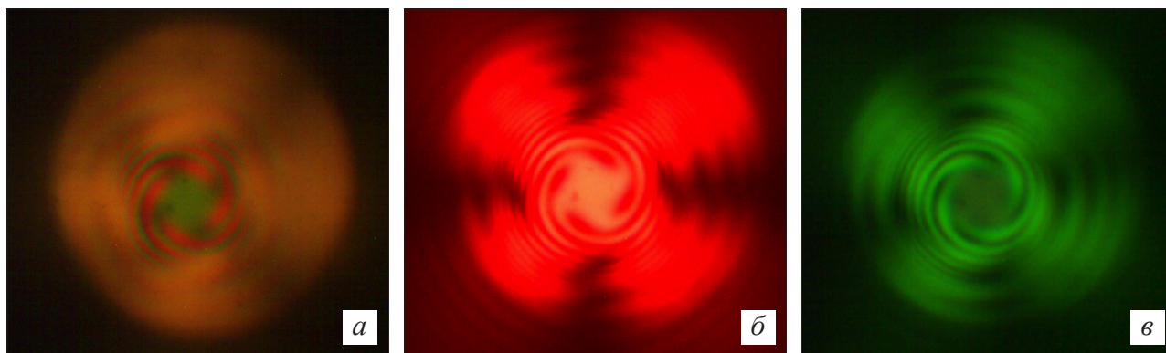
Рис. 4. Вид спиралей Эри в отсутствии светофильтров (а), со светофильтрами КС10 (б) и ЗС1 (в)
