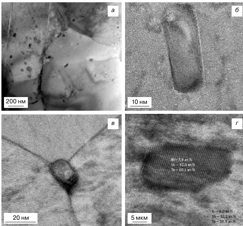
Рис. 8. Светлопольные изображения структуры термоэлектрического материала состава \text{Bi}_{0,4}\text{Sb}_{1,6}\text{Te}_3 , полученного методом SPS при температуре 450 °С: а — наночастицы в зернах образца; б, в — изображение высокого разрешения наночастицы в объеме зерна на стыке трех зерен; г — сравнение составов твердого раствора в наночастице и окружающем зерне, определенных методом локального энергодисперсионного анализа
