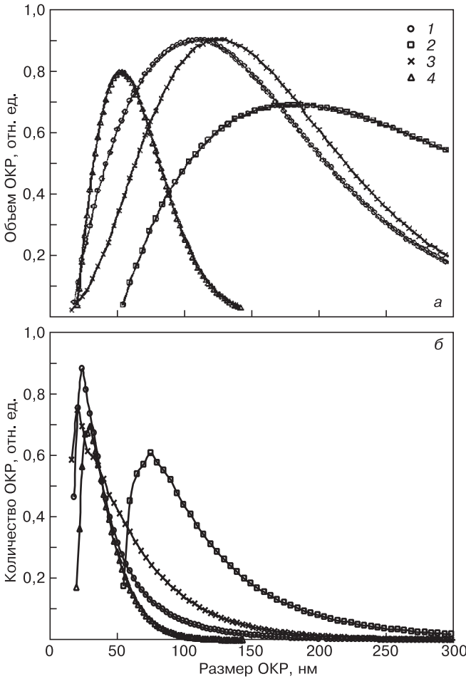
Рис. 3. Зависимости объема (а) и количества (б) ОКР от их размера в образцах Bi_{0,4}Sb_{1,6}Te_3 , полученных спеканием при различных температурах T_{SPS} , °С: 1 — 250; 2 — 300; 3 — 450; 4 — 500
