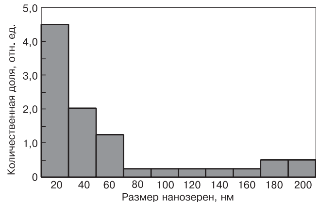
Рис. 4. Гистограмма распределения количественной доли нанозерен по их размерам в компактном наноструктурированном образце Bi_{0,5}Sb_{1,5}Te_3 по данным работы [22]
