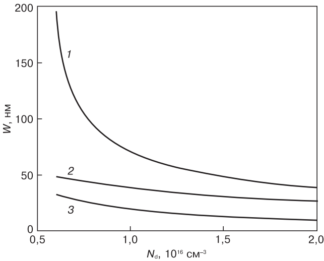
Рис. 4. Зависимости ширины потенциального барьера от концентрации доноров для кристаллита с параметрами T = 300 \text{ К} , \epsilon = 10 , R = 600 \text{ нм} , N_s = 10^{11} \text{ см}^{-2} . Цифрами обозначено: 1 — численный расчет; 2 — оценка по модели Seto; 3 — длина Дебая
