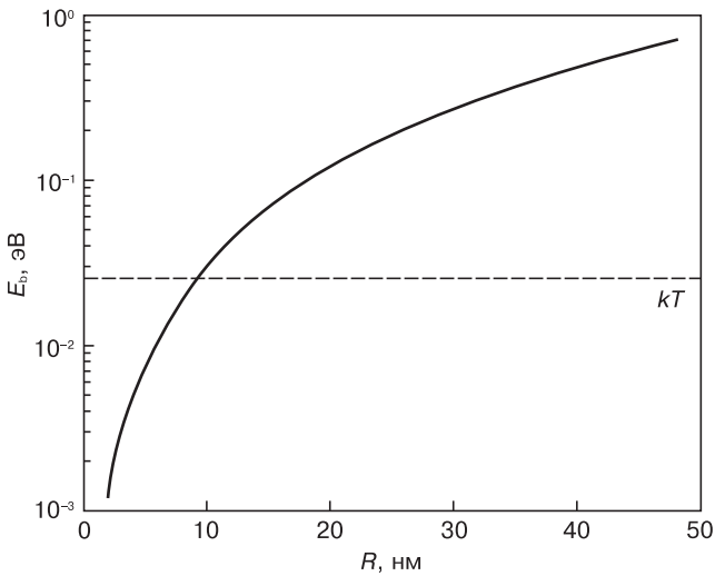
Рис. 3. Зависимость максимальной высоты потенциального барьера от радиуса сферического кристаллита ( N_d = 10^{18} \text{ см}^{-3} , T = 300 \text{ К} и \epsilon = 10 ). Пунктир — величина kT
